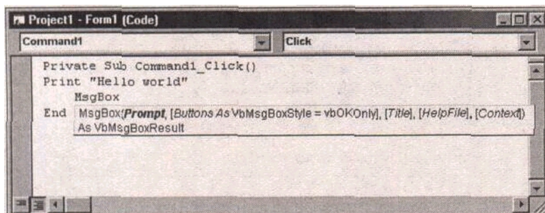
Рис. 1.19. Отображение синтаксиса оператора в подсказке
