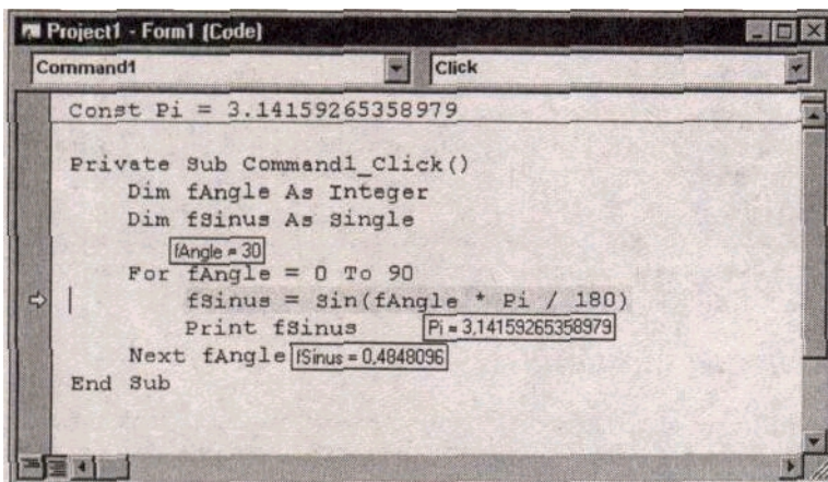
Рис. 5.20. Пример Data Tips для различных переменных
