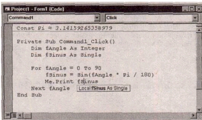
Рис. 5.21. Результат вызова команды Edit\QuickInfo для переменной
