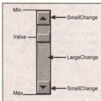
Рис. 3.4. Различные свойства полос прокрутки
