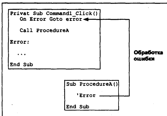
Рис. 5.7. Обработка ошибок во вложенных процедурах
