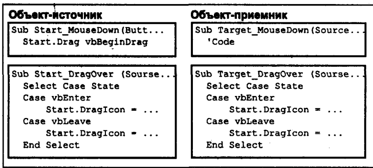
Рис. 10.4. Процесс перетаскивания с меняющимся курсором мыши
