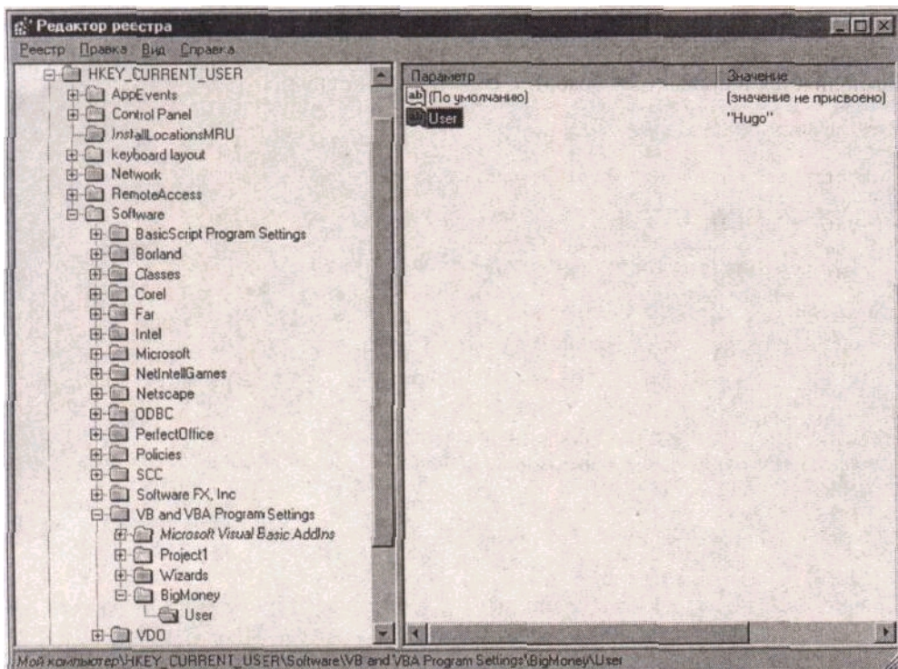
Рис. 2.8. Установки реестра и их сохранение
