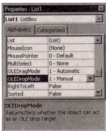
Рис. 10.8. OLEDragMode и OLEDropMode в окне свойств
