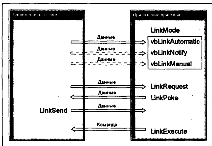
Рис. 6.8. Обобщение свойств и методов DDE
