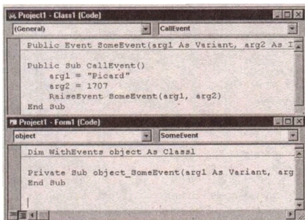
Рис. 7.12. Событие, определяемое пользователем
