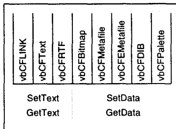
Рис. 6.3. Структура объекта Clipboard
