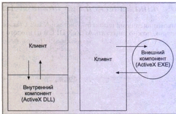
Рис. 8.18. Клиенты и компоненты
