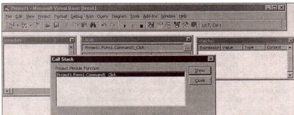
Рис. 5.26. Окна режима отладки
