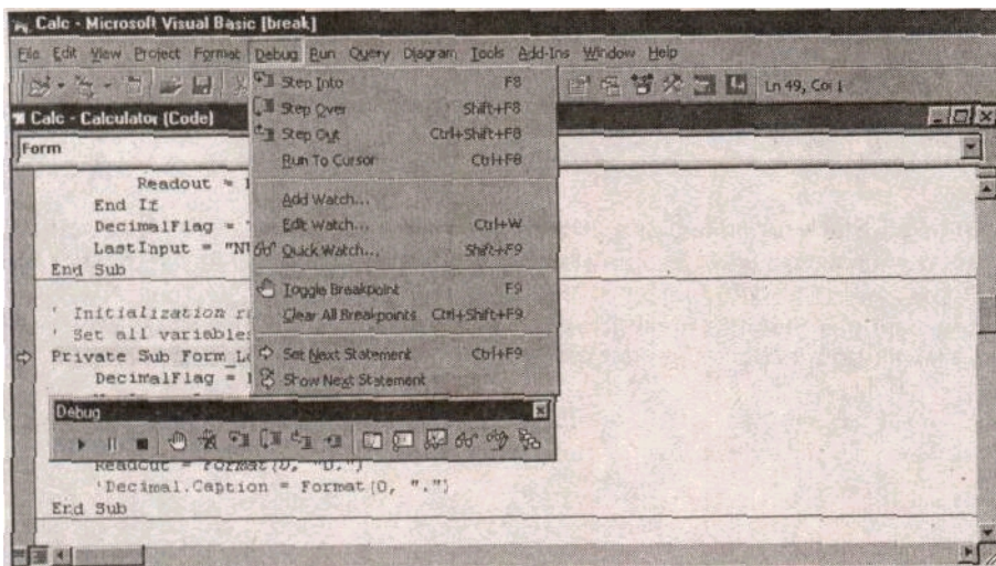
Рис. 5.19. Инструменты для контроля выражений
