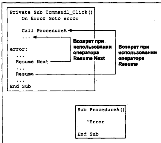
Рис. 5.8. Возврат при обработке ошибок во вложенных процедурах
