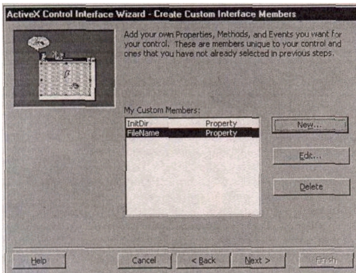
Рис. 8.5. Окно мастера интерфейсов. Этап 2
