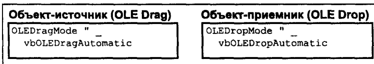
Рис. 10.7. Установка автоматического режима OLEDragMode и OLEDropMode
