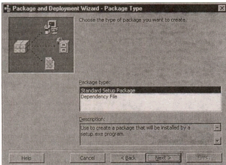
Рис. 10.23. Мастер установки
