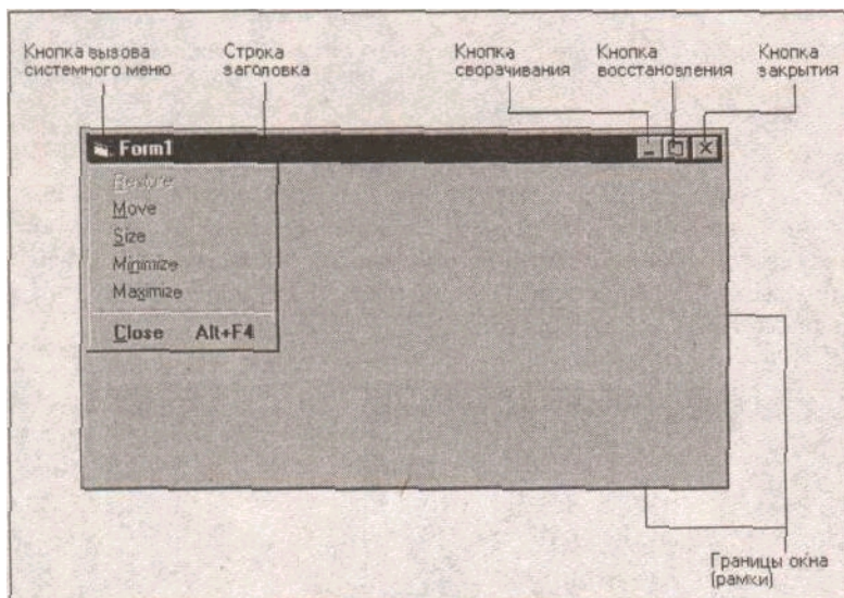
Рис. 3.2. Элементы окна
