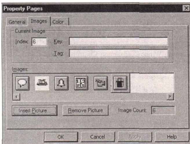
Рис. 1.1. Свойства ImageList
