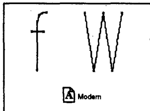
Рис. 4.11. Векторный шрифт
