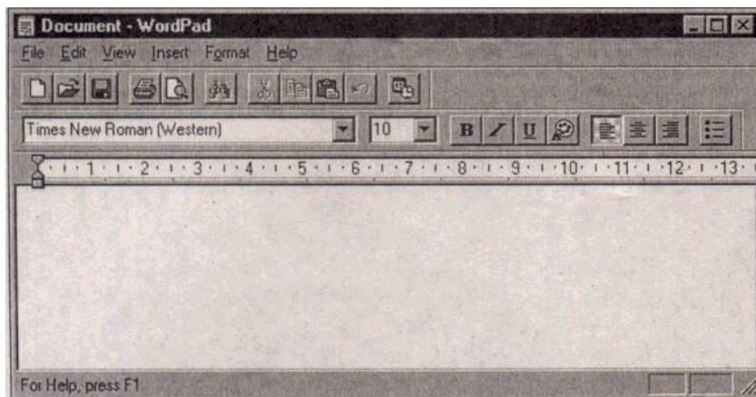
Рис. 10.20. Microsoft WordPad
