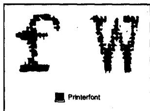
Рис. 4.13. Принтерный шрифт
