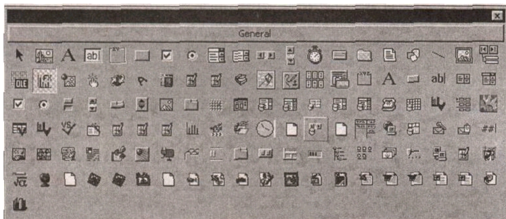
Рис. 1.9. Панель элементов
