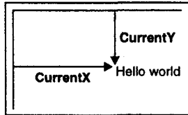
Рис. 4.15. Позиция печати
