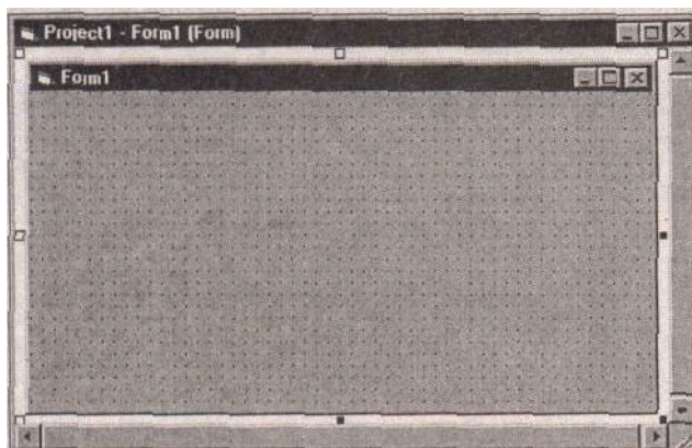
Рис. 1.10. Окно формы
