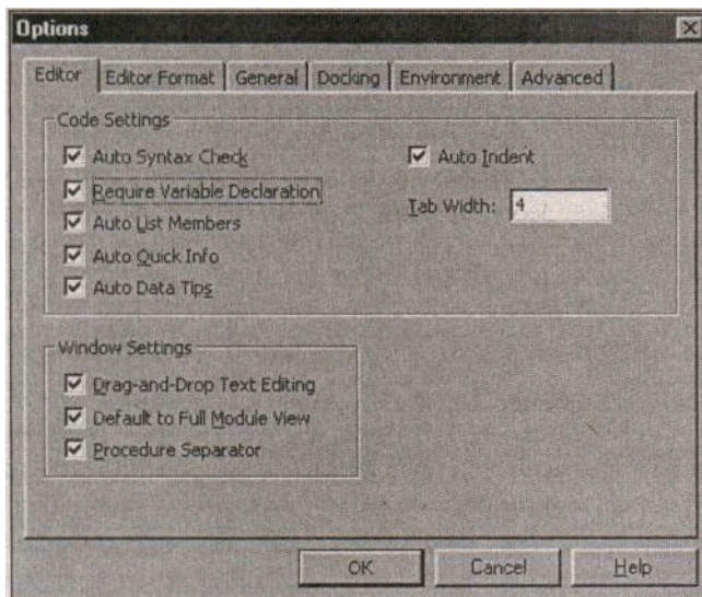
Л/с 5.3(i). Установки Require Variable Declaration
