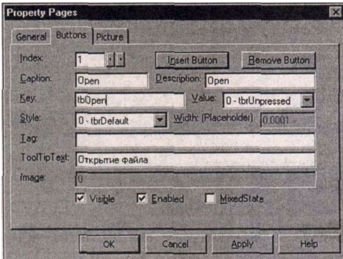
Рис. 3.9. Свойства элемента управления ToolBar
