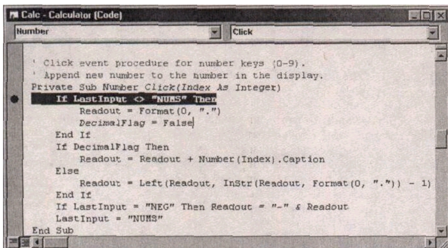
Рис. 5.13. Строка с точкой останова в окне кода
