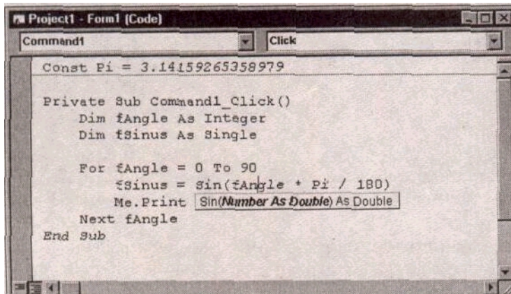
Рис. 5.22. Результат выполнения команды Edit\Parameter Info параметра
