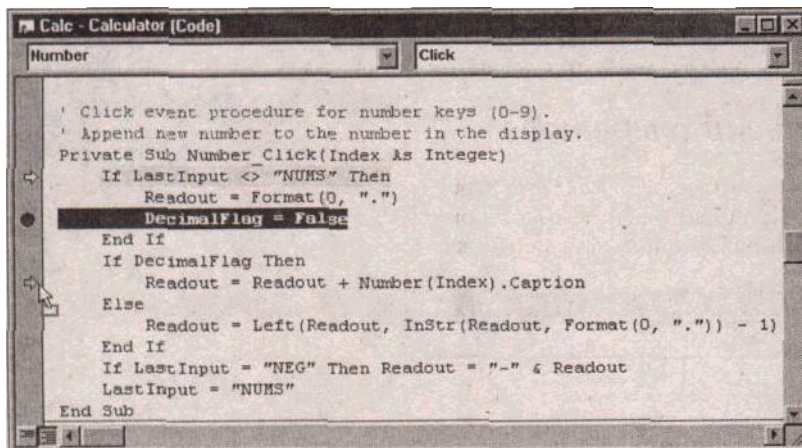
Рис. 5.1?. Перемещение маркирования для следующей строки выполнения
