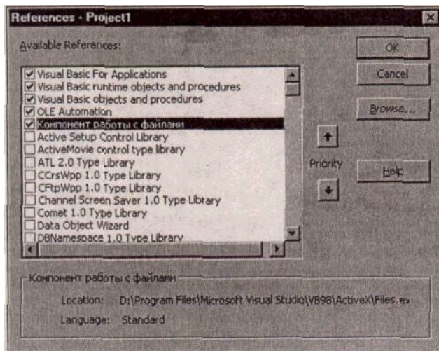
Рис. 8.14. Диалоговое окно References
