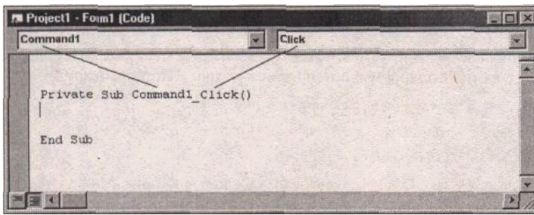
Рис. 1.23. Структура имени процедуры
