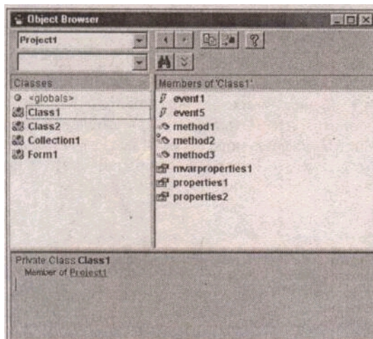
Рис. 7.14. Каталог объектов с классом, определяемым пользователем
