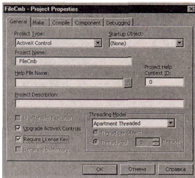
Рис. 8.14. окно Project Properties
