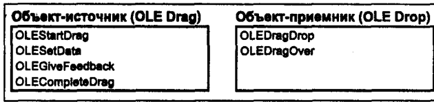
Рис. 11.9. События при перетаскивании с использованием OLE
