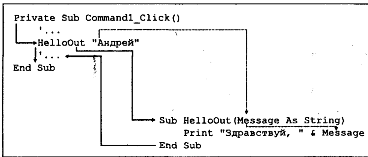
Рис. 1.26. Вызов процедуры с аргументом
