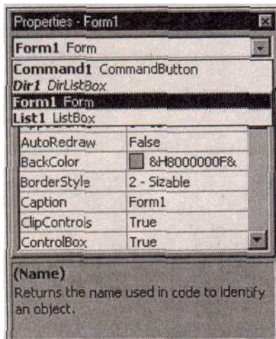
Рис. 10.5. Типы элементов управления в окне свойств
