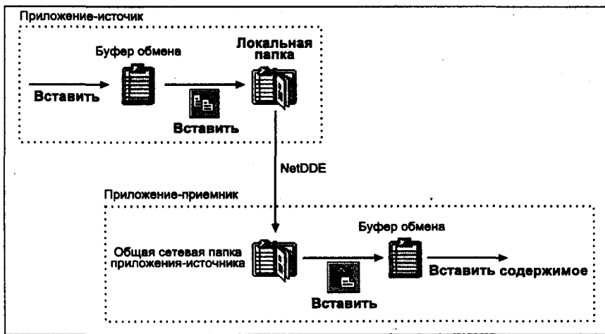
Рис. 6.6. NetDDE-связь через папку для обмена
