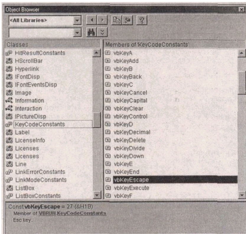
Рис. 4.9. Константы клавиатуры в каталоге объектов
