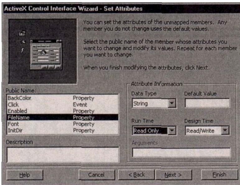
Рис. 8.7. Окно мастера интерфейсов. Этап 4
