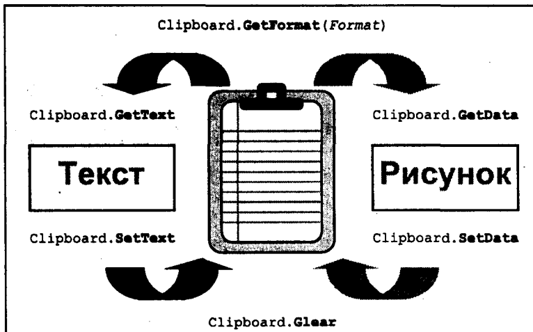
Рис. 6.2. Методы объекта Clipboard
