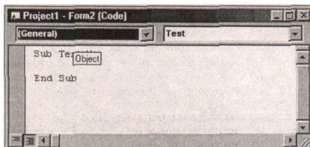
Рис. 2.4. Общие процедуры в окне кода
