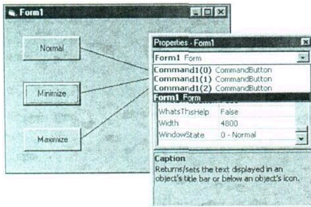
Рис. 2.7. Пример массива элементов управления
