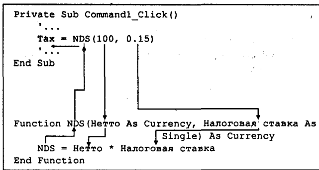
Рис. 1.27. Вызов функции с аргументами
