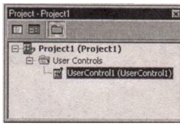
Рис. 8.2. Структура проекта
