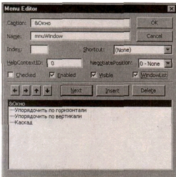
Рис. 10.19 Редактор меню
