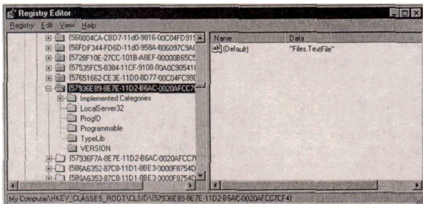
Рис. 25. Запись реестра
