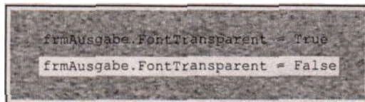
Рис. 4.14. Свойство FontTransparent
