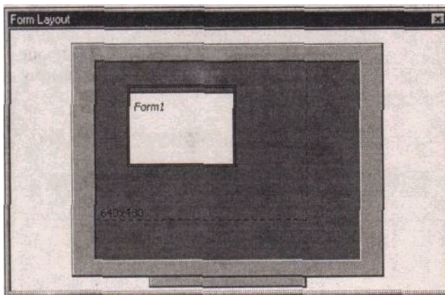
Рис. 1.15. Раскладка башка
