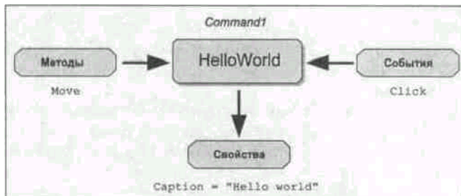
Рис. 1.21. Категории объектов
