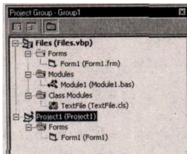
Рис. 8.20. Группа проектов
