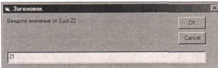
Рис. 4.4. Окно InputBoa
