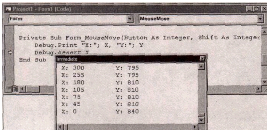
Рис. 5.33. Метод Assert
