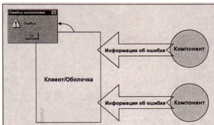
Рис. 8.16. Ошибка выполнения
