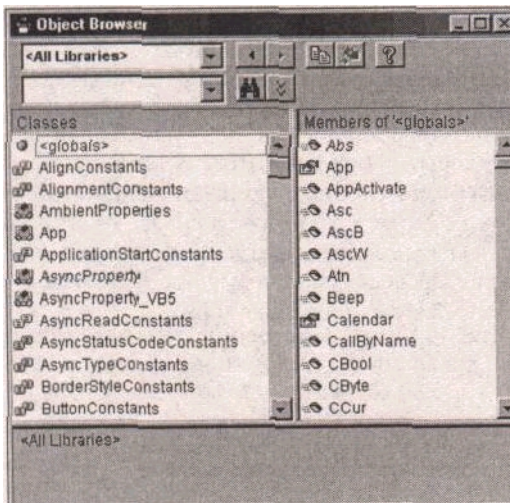
Рис. 1.24. Каталог объектов
