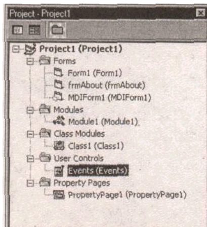
Рис. 1.12. Окно проекта
