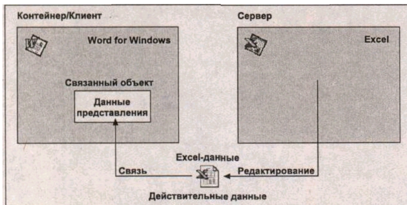
Рис. 8.3. Связанные объекты
