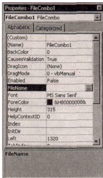
Рис. 8.11. Свойства FileCombo
