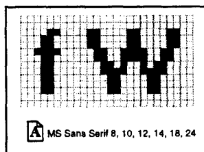
Рис. 4.10. Растровый шрифт
