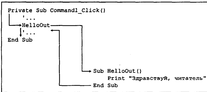
Рис. 1.25. Вызов процедуры
