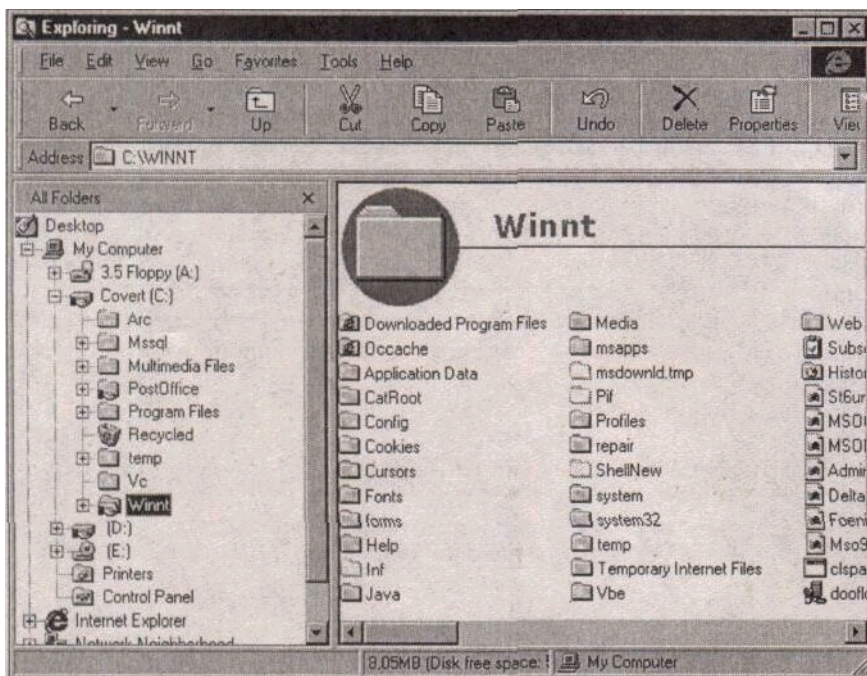
Рис. 10.21. Проводник Windows
