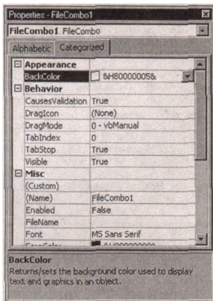
Рис. 8.13. Категории свойств
