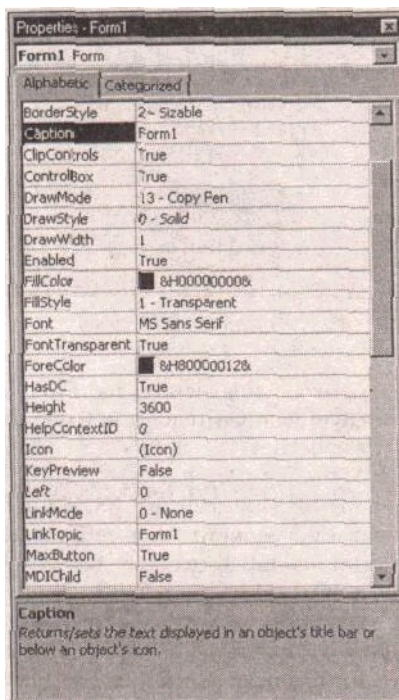
Рис. 1. 11. Окно свойств
