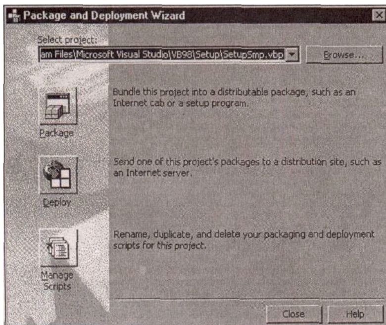
Рис. 10.22. Мастер инсталляции
