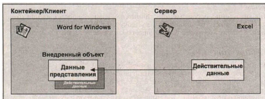
Рис. 8.2. Данные представления и естественные данные
