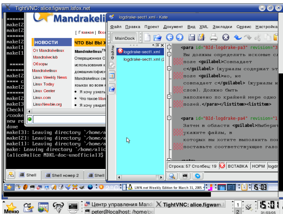
Рисунок 2-4. Управление удалённым компьютером
