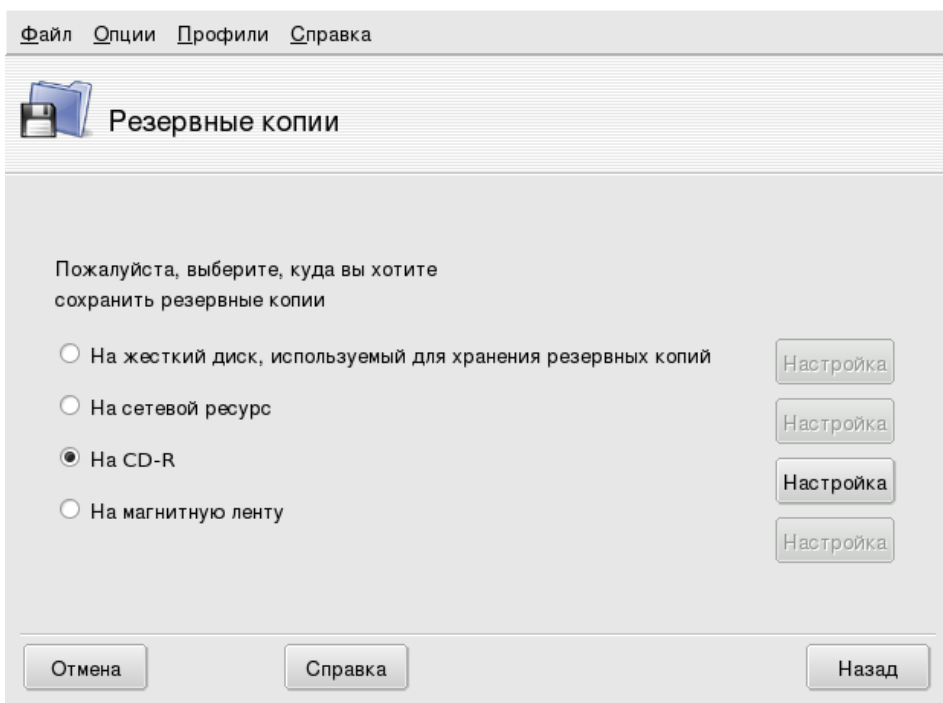
Рисунок 5-17. Выбор места хранения резервной копии
