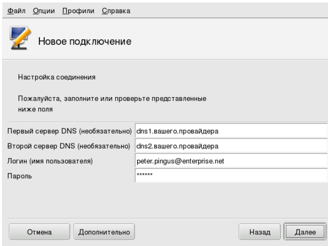
Рисунок 4-4. Настройка параметров подключения ADSL
