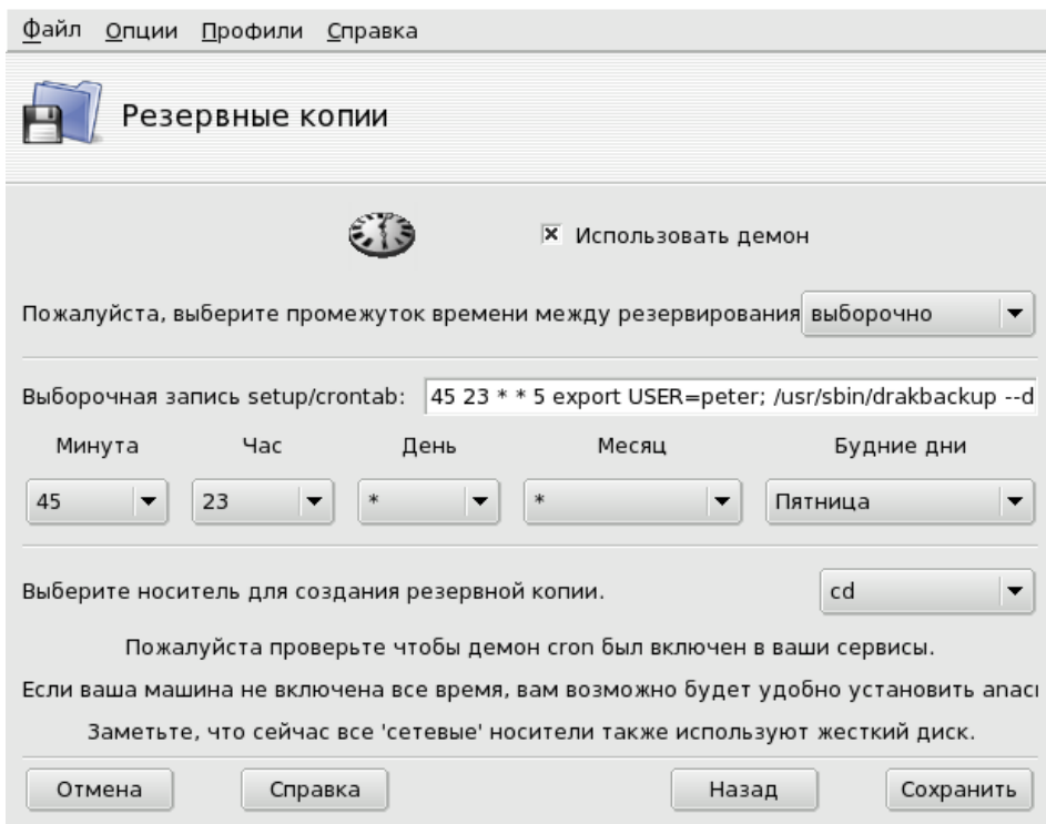
Рисунок 5-21. Окно параметров демона
