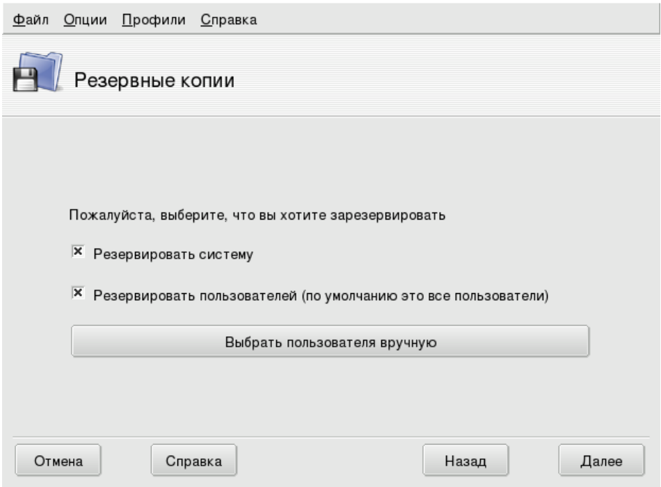
Рисунок 5-16. Выбор резервируемых данных
