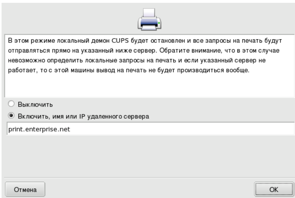
Рисунок 3-14. Настройка режима клиента
