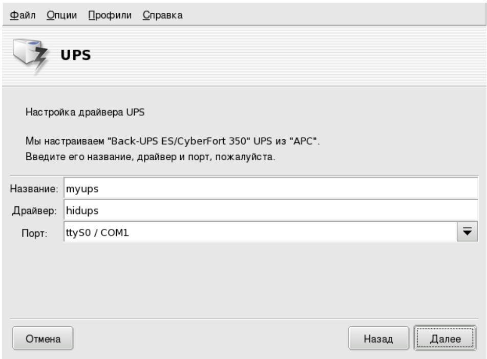
Figure 3-31. Название, устройство и порт
