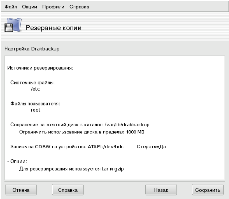
Рисунок 5-19. Просмотр конфигурационных параметров
