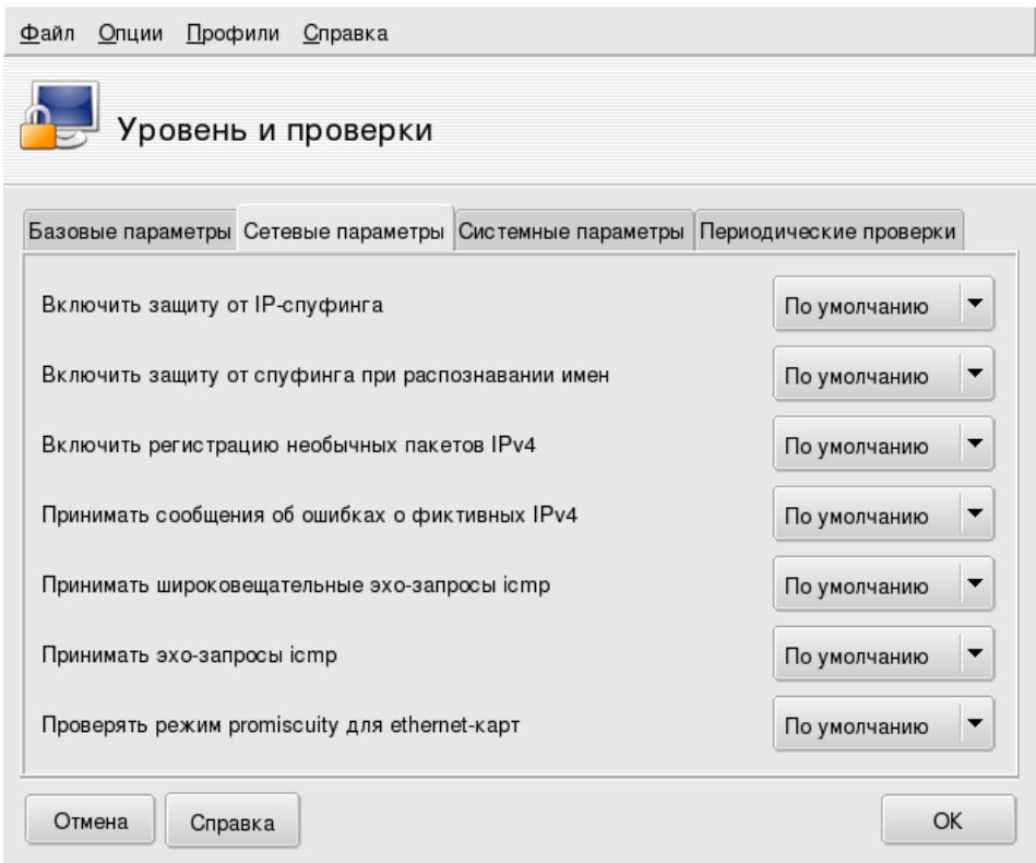
Рисунок 7-2. Изменение стандартных параметров
