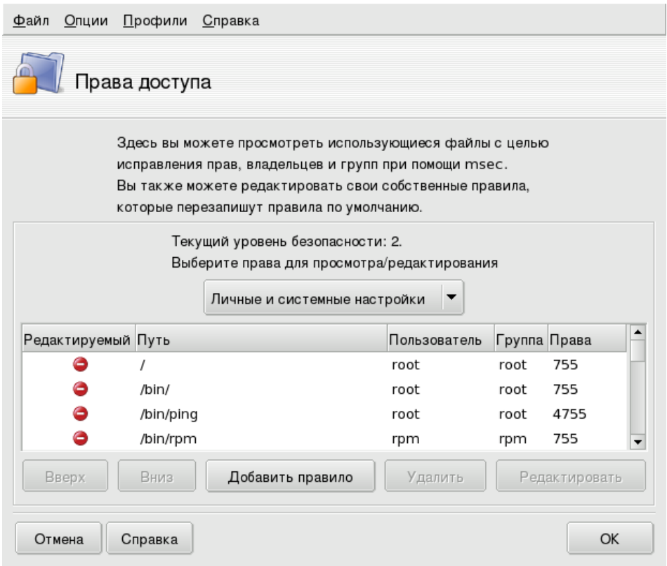
Рисунок 7-3. Настройка проверки прав доступа к файлам
