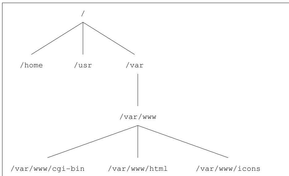
Рисунок 6-3. Файловая система теперь примонтирована
