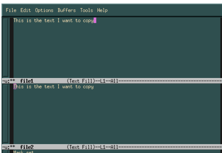
Рисунок 8-3. Копирование текста в emacs
