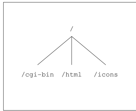
Файловая система, содержащая файлы каталога "/var/www" (ещё не примонтирована)
